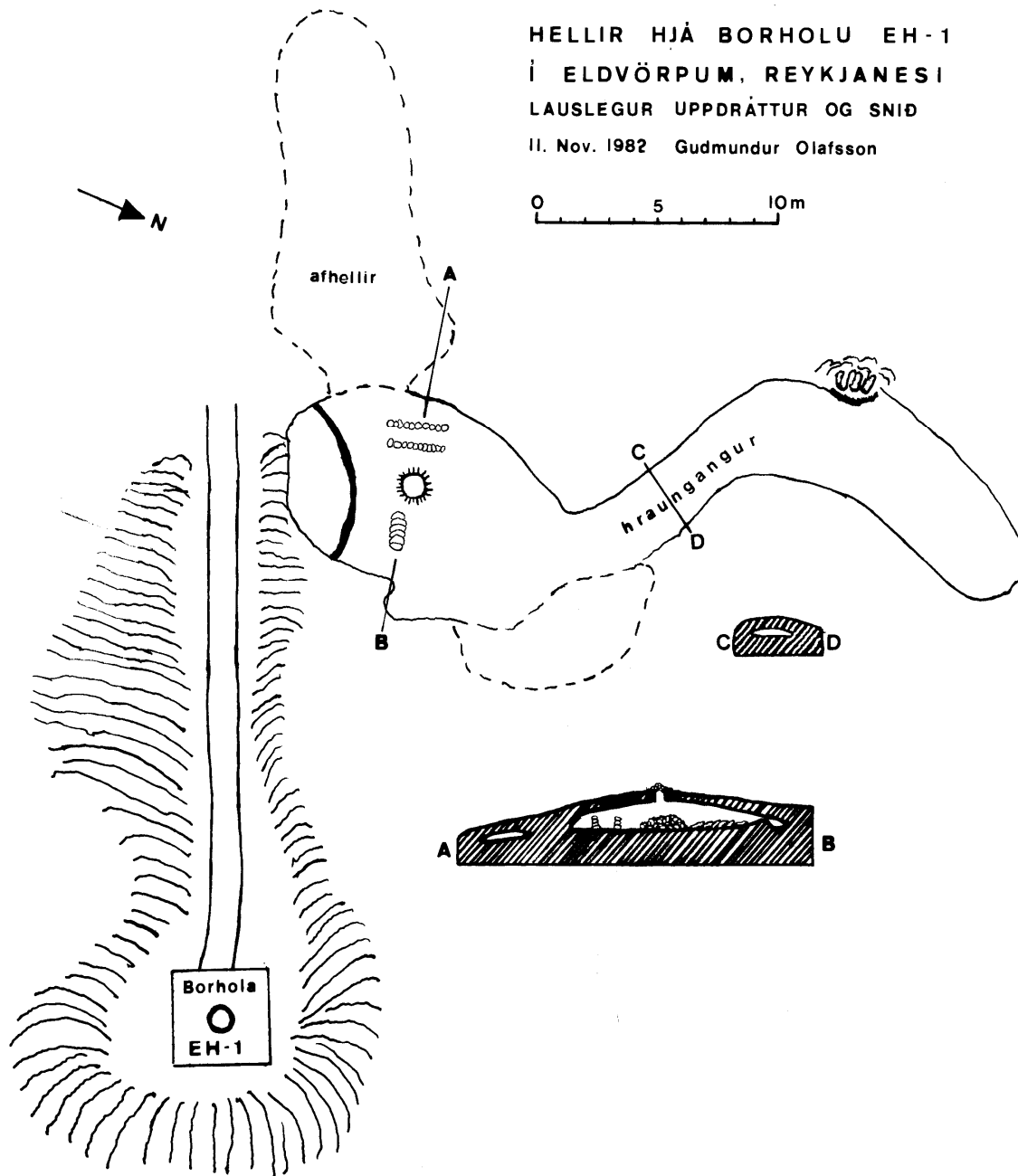
Mynd 4. Flatarteikning og sniðteikningar af hellinum og afstaða hans við borholu (Teikn. GÓ.).
