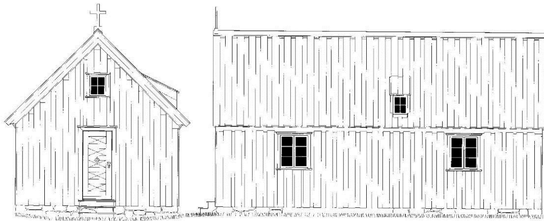
Sjávarborgarkirkja, þverskurður, langskurður, grunnmynd og útlit. Teikningar arkitektanna Grétars Markússonar og Stefáns Arnar Stefánssonar.
